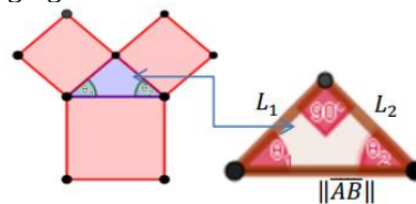
Gambar 2. Segitiga Siku-Siku
