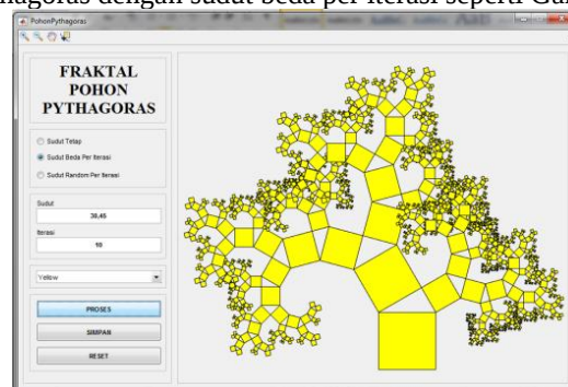
Gambar 9. Iterasi ke-10 dan Sudut \theta = 30^\circ, 45^\circ pada Aturan Sudut Beda Per Iterasi
