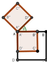
Gambar 5. Persegi yang Didilatasi dan Dirotasi
