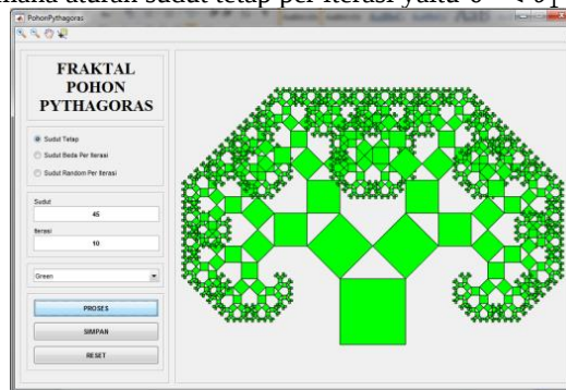
Gambar 8. Iterasi ke-10 dan Sudut \theta = 45^\circ pada Aturan Sudut Tetap
