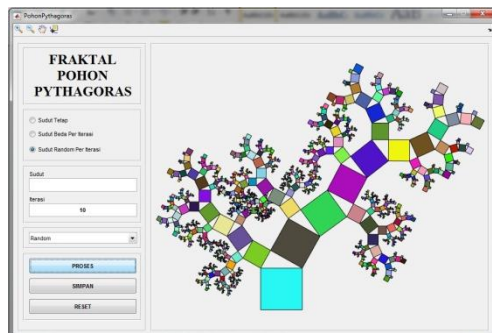
Gambar 10. Iterasi ke-10 pada Aturan Sudut Random Per Iterasi
