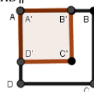
Gambar 3. Persegi yang Didilatasi dengan Pusat A(x, y)
