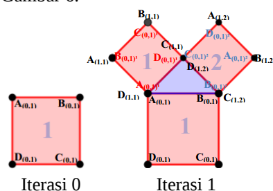
Gambar 6. Visualisasi Pembentukan Pohon Pythagoras dari Iterasi 0 ke 1
